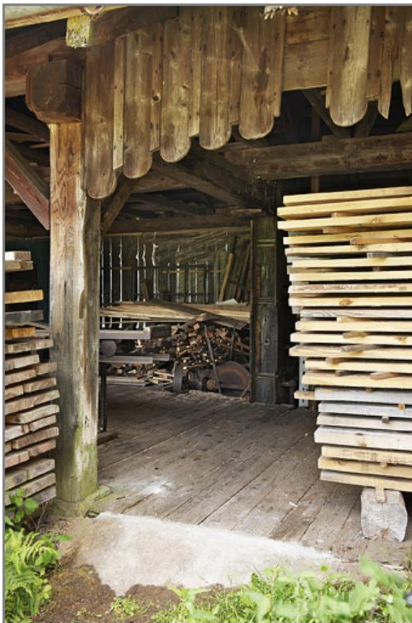
Les Rouges-Eaux, scierie du Pré-Laurent, halle de sciage.
